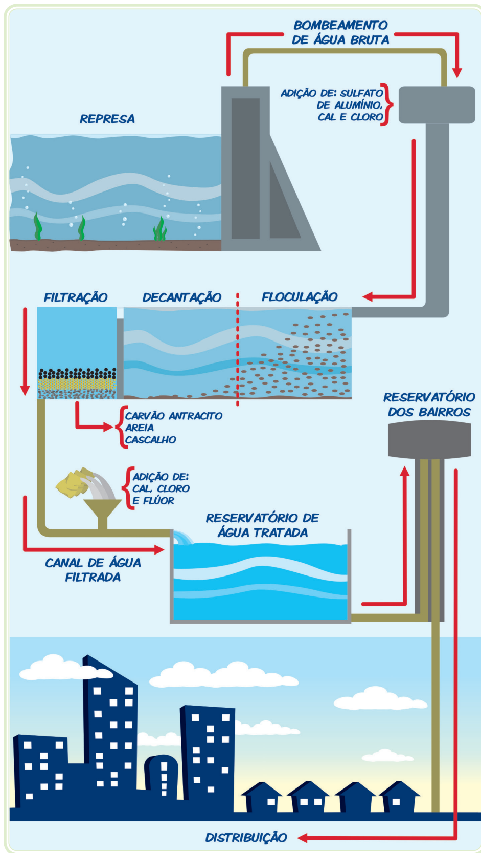
Figura 4.1: Tratamento de água Fonte: CTISM
