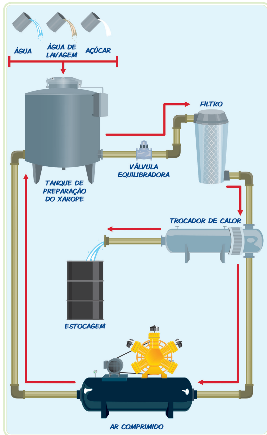
Figura 4.3: Preparação de xarope de açúcar em indústrias de bebidas
