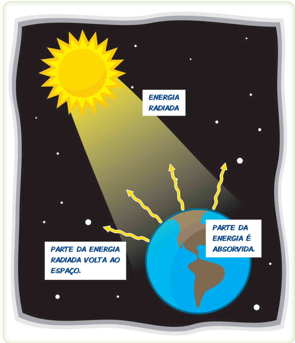
Figura 2.1: Efeito estufa
