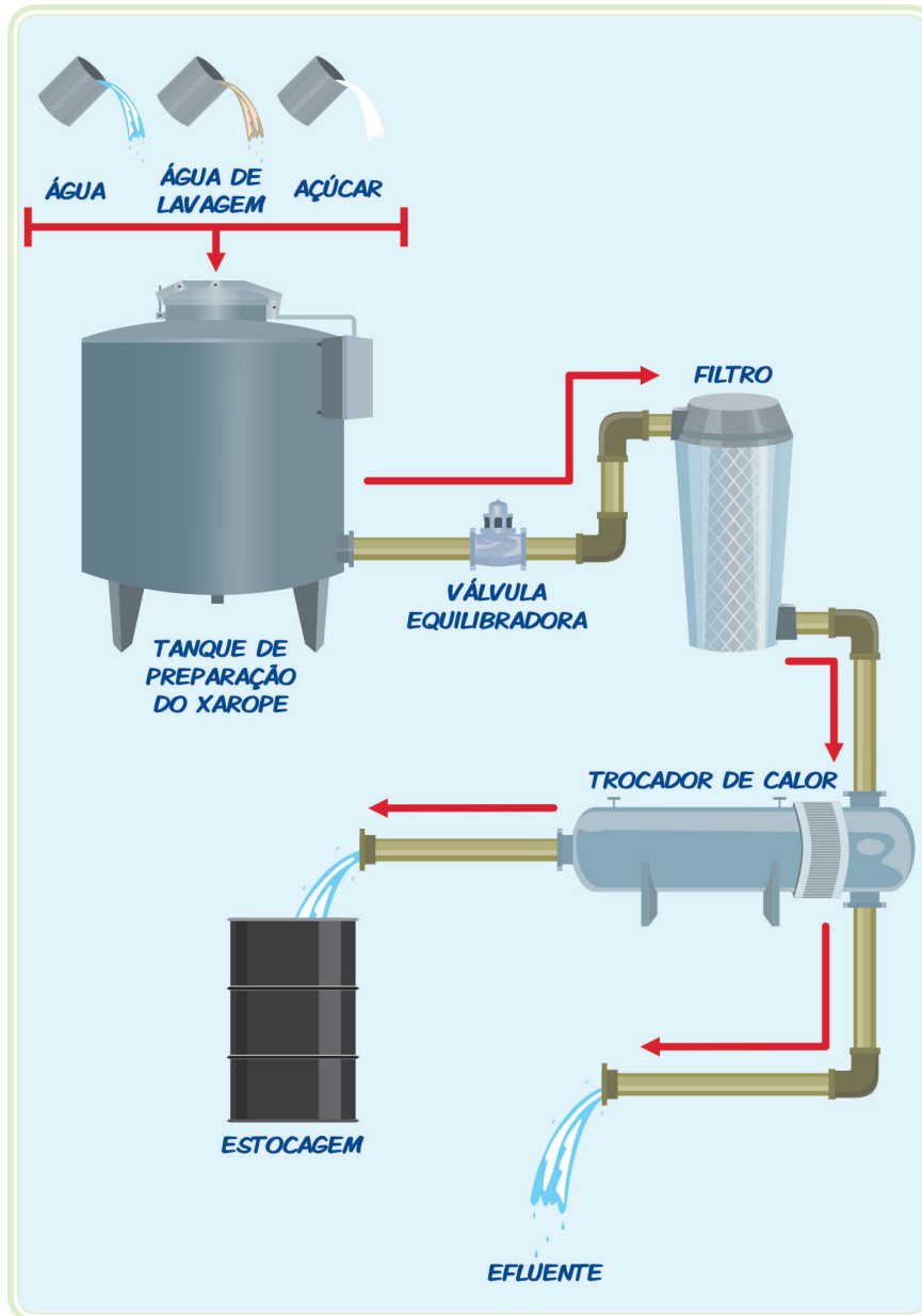
Figura 4.2: Preparação de xarope de açúcar em indústrias de bebidas
